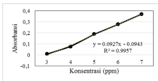
Gambar 1. Kurva Baku Larutan Vitamin C
